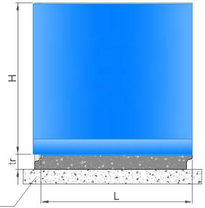
SEZIONE LONGITUDINALE
