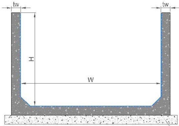
SEZIONE TRASVERSALE
